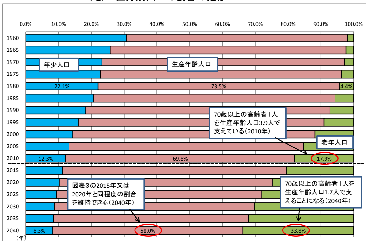
図表7 生産年齢人口を15歳以上70歳未満と仮定した場合の年齢3区分別人口の割合の推移
