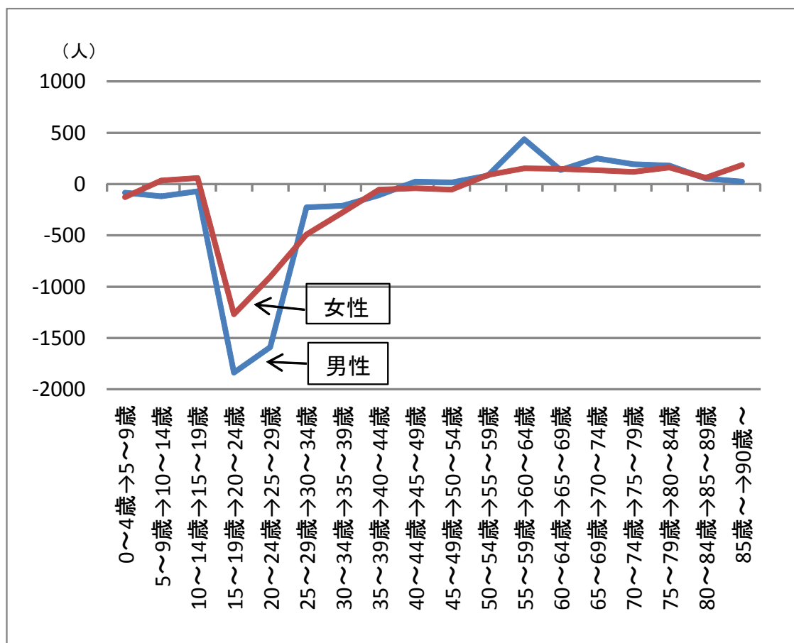
図表14 2005（平成17）年→2010（平成22）年の年齢階級別人口移動
