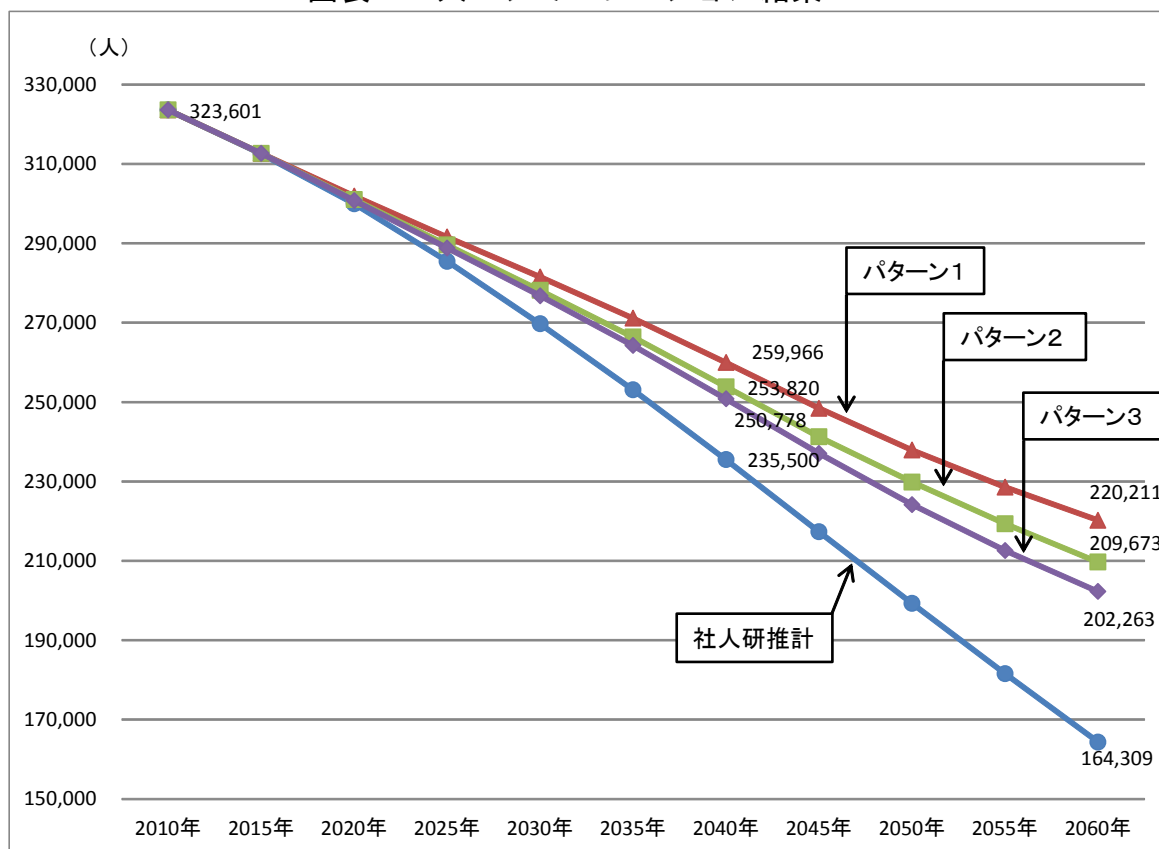
図表51 人口シミュレーション結果
