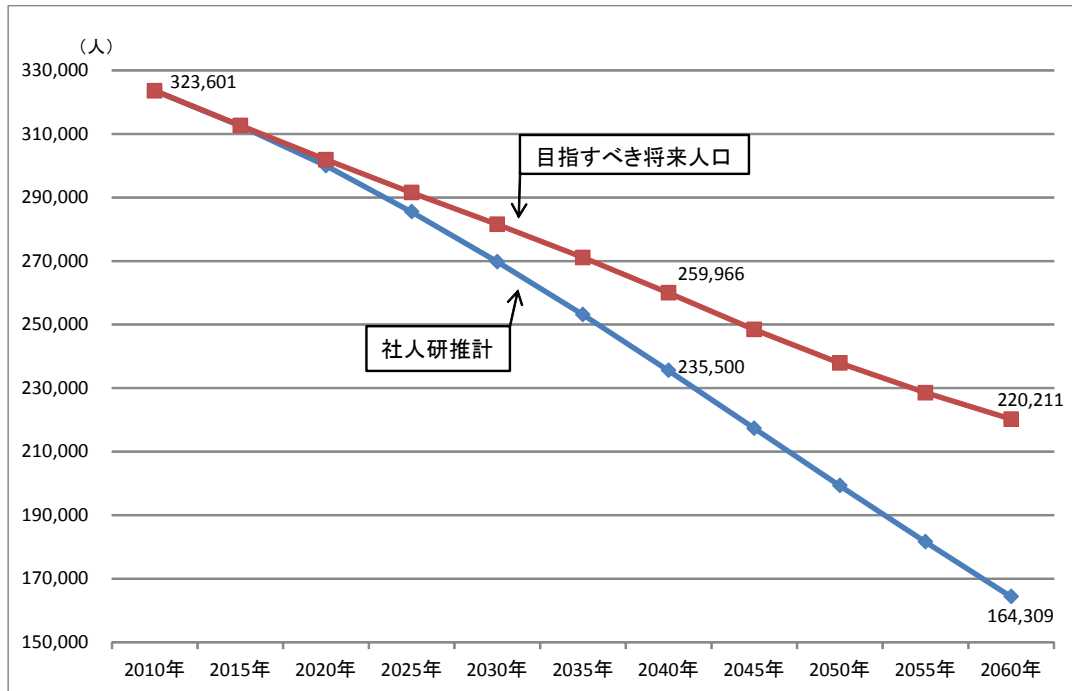
図表52 目指すべき将来人口
