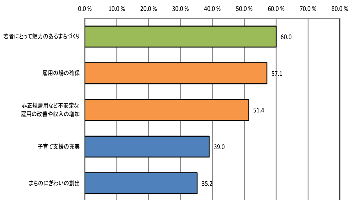
図表48 調査結果：秋田市に住み続けるために必要なこと【20代】
