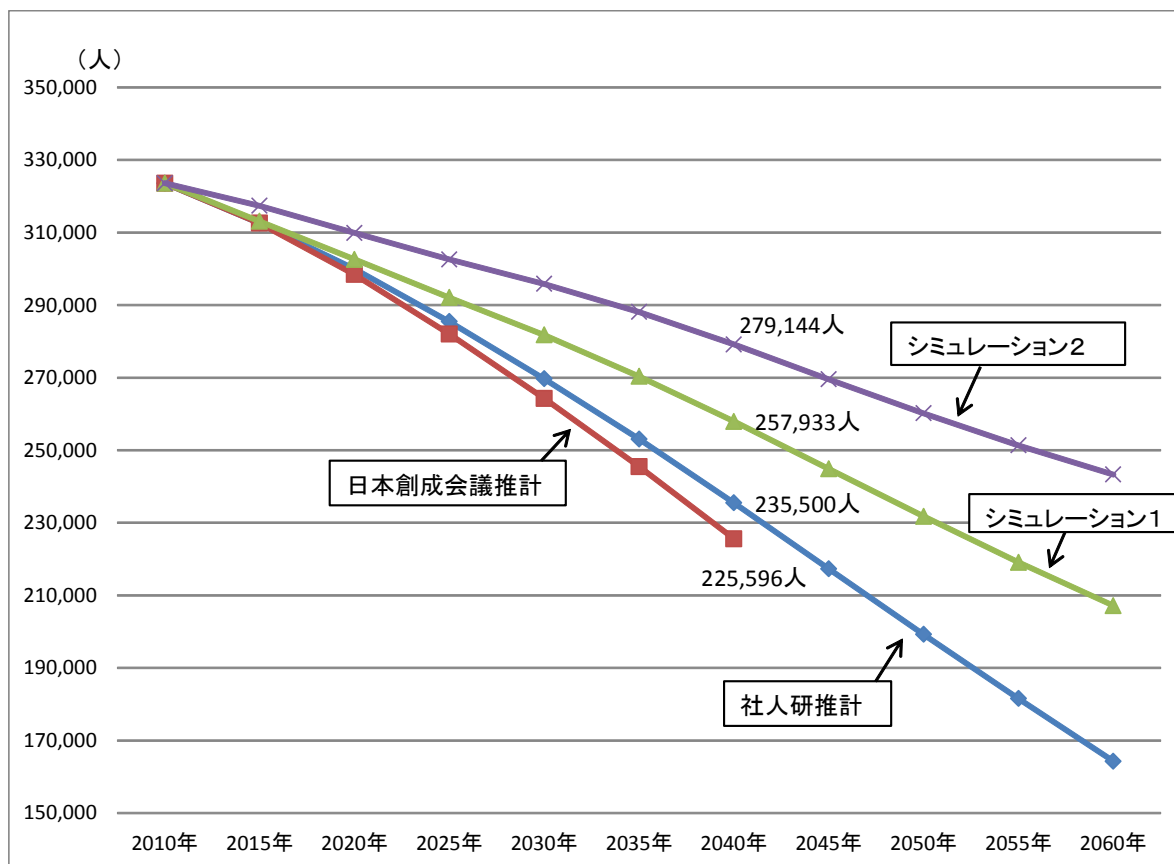
図表23 総人口の推計結果（社人研推計・日本創成会議推計・シミュレーション1、2）
