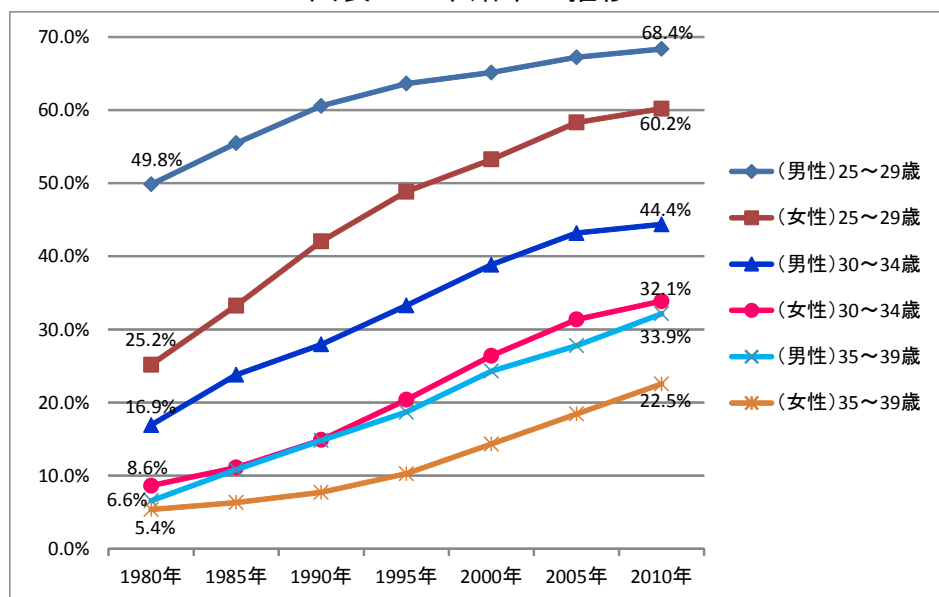
図表11 未婚率の推移
