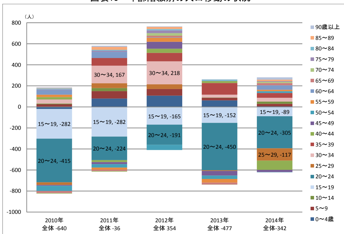
図表13 年齢階級別の人口移動の状況
