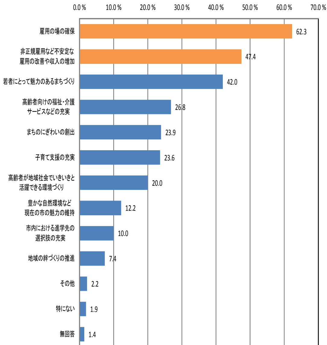
図表46 調査結果：秋田市に住み続けるために必要なこと（全体）
