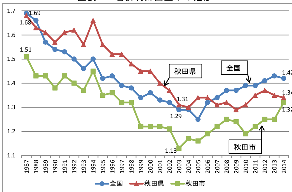
図表10 合計特殊出生率の推移
