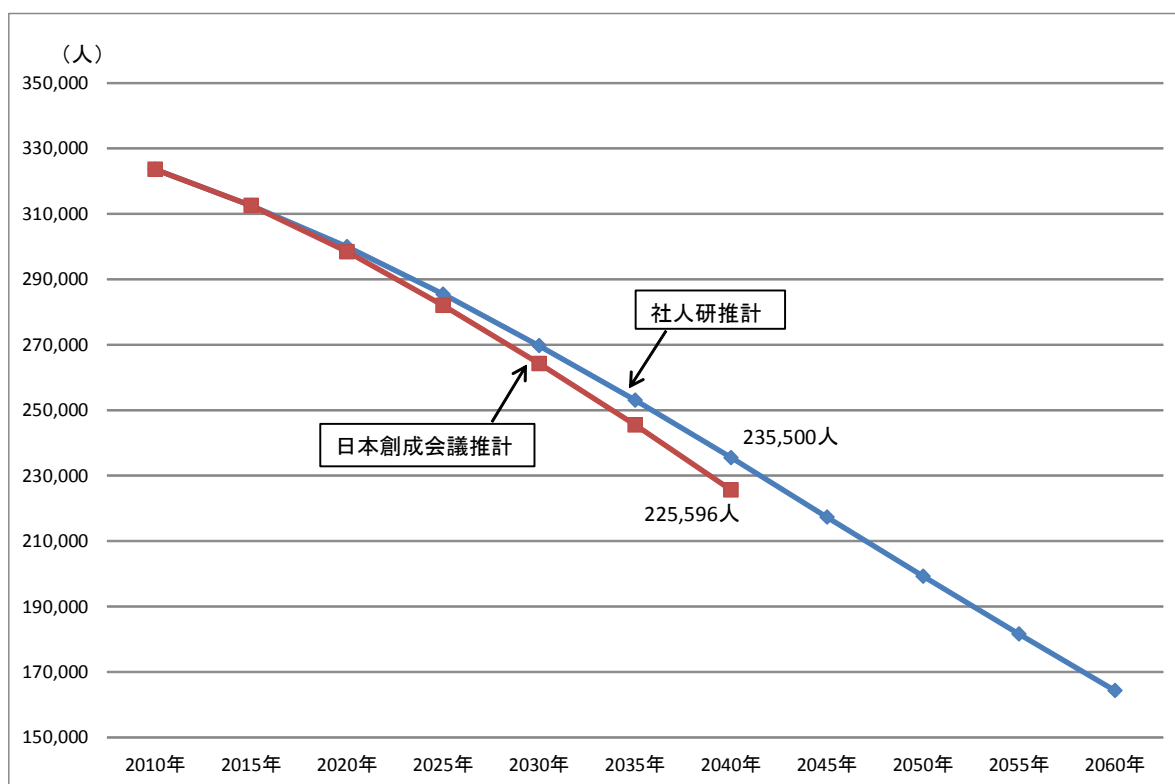
図表21 社人研推計と日本創成会議推計との総人口の比較
