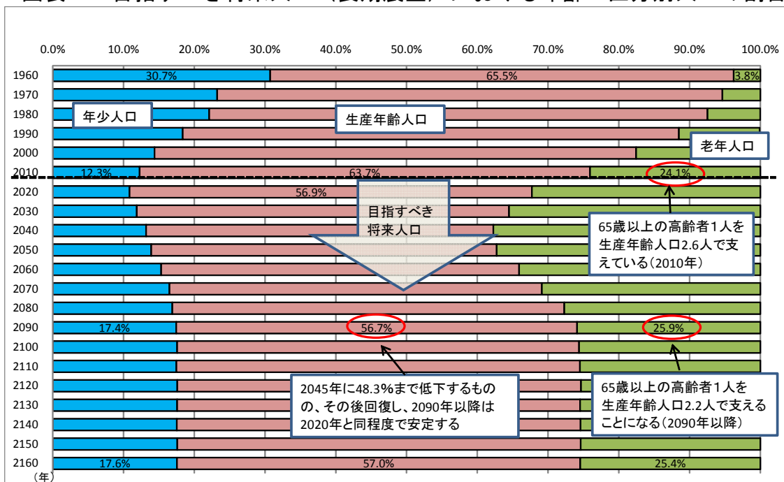
図表54 目指すべき将来人口（長期展望）における年齢3区分別人口の割合
