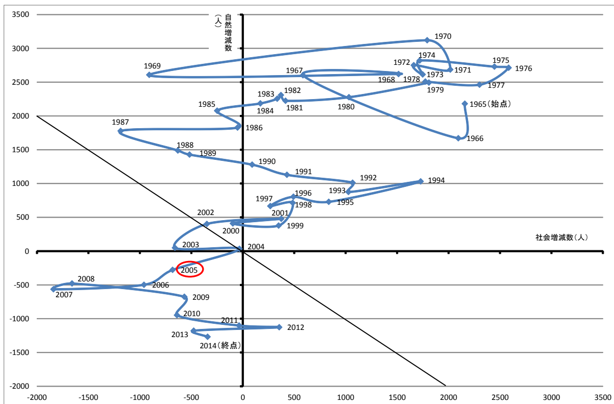
図表9 総人口の推移に与えてきた自然増減と社会増減の影響
