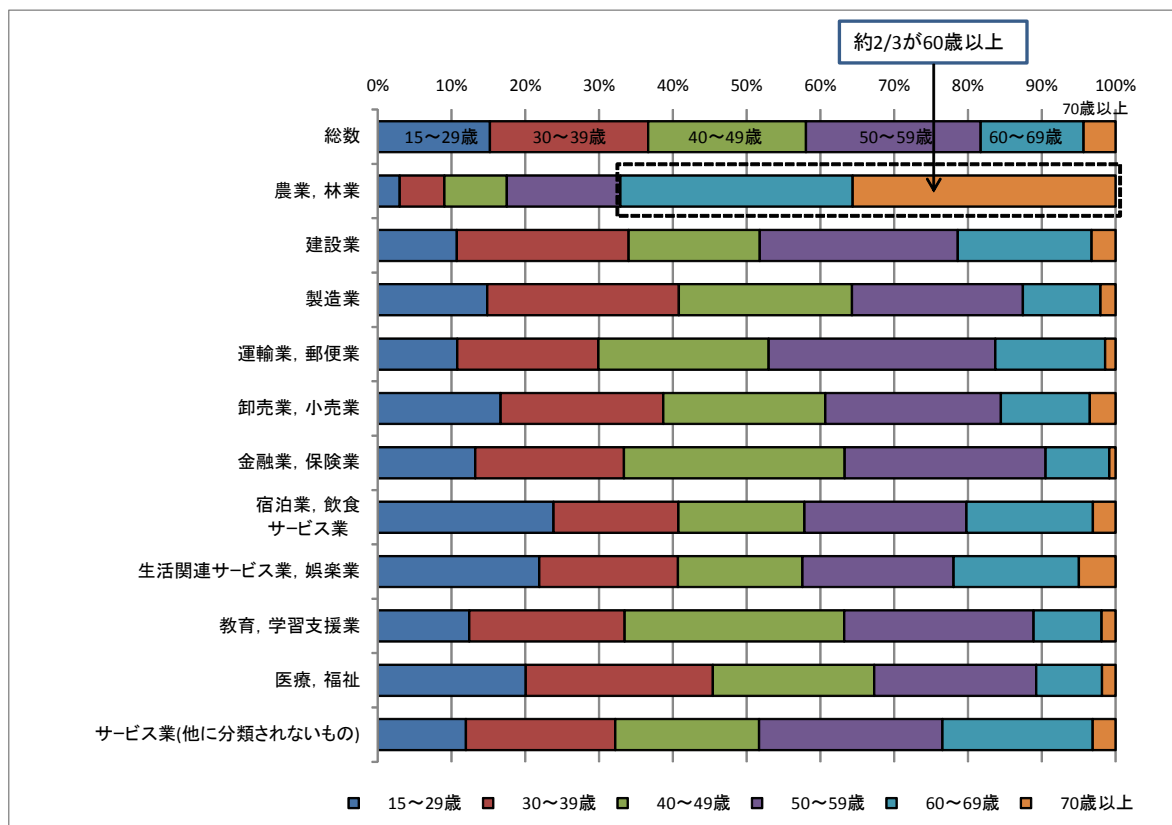
図表20 産業別年齢構成
