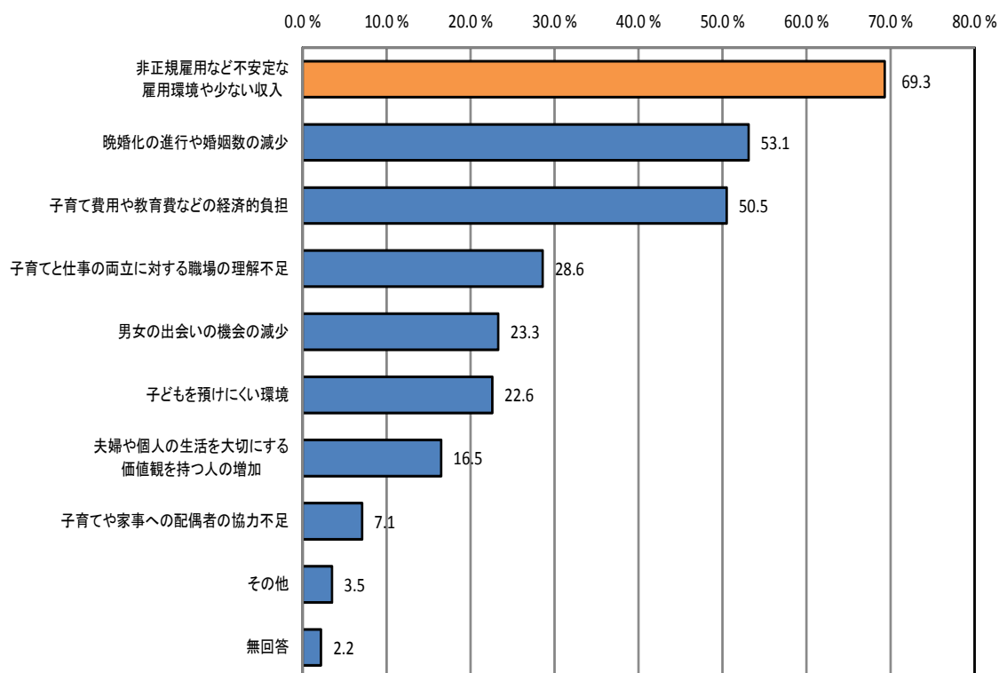
図表44 影響が大きい少子化要因（全体）
