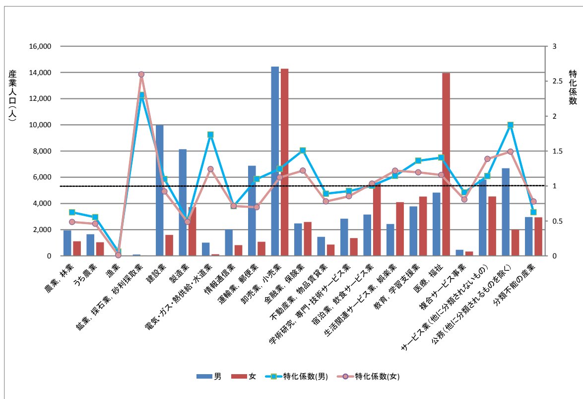
図表19 男女別産業人口
