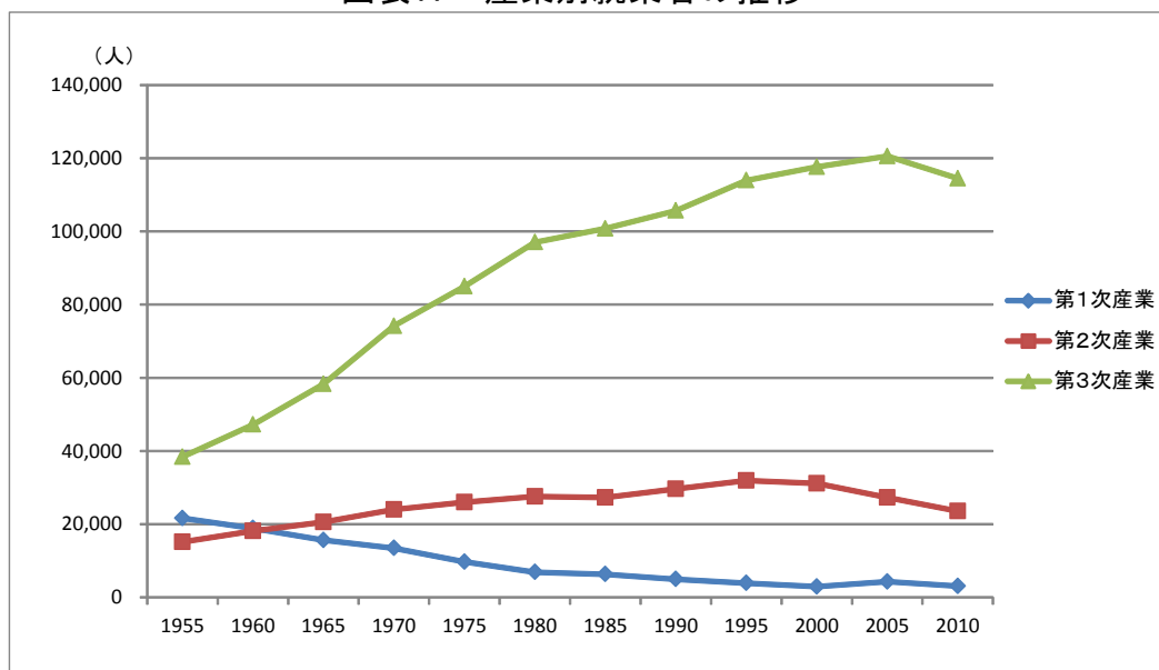
図表17 産業別就業者の推移
