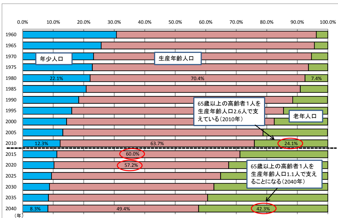
図表3 年齢3区分別人口の割合の推移
