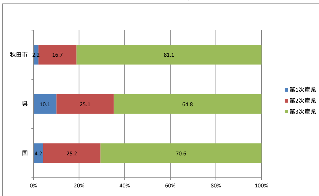
図表18 産業別就業者構成比
