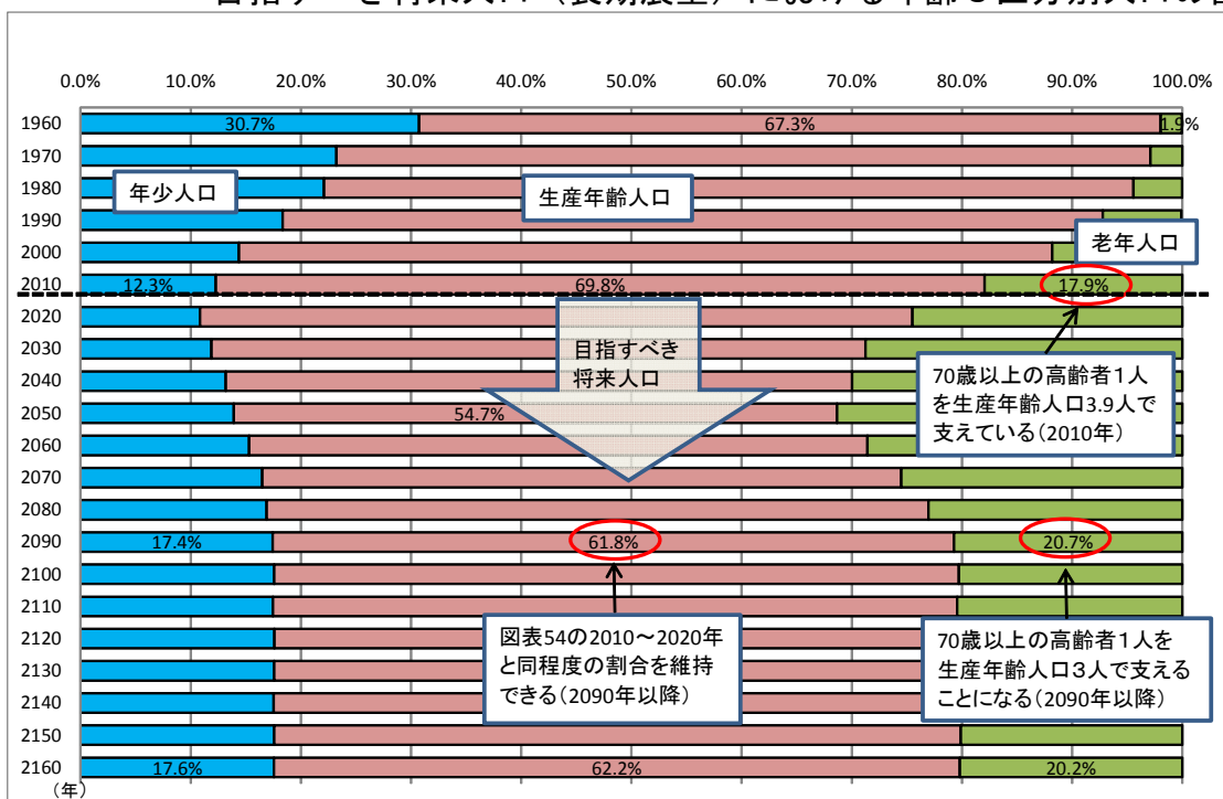
図表55 生産年齢人口を15歳以上70歳未満と仮定した場合の 目指すべき将来人口（長期展望）における年齢3区分別人口の割合
