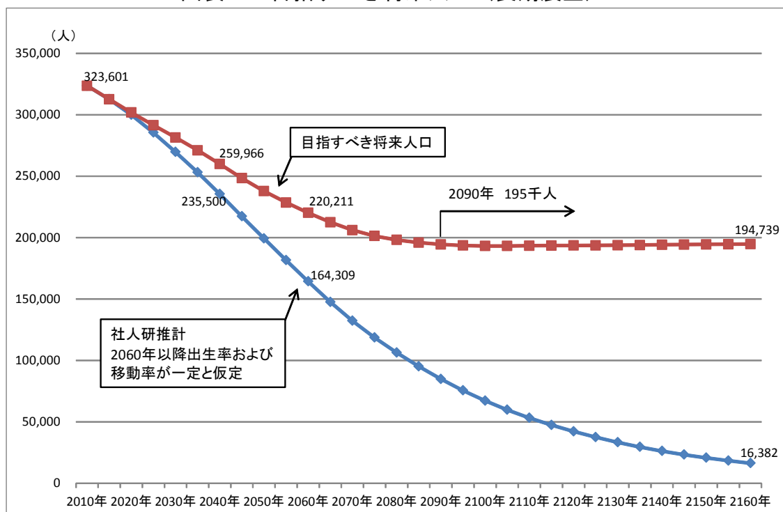
図表53 目指すべき将来人口（長期展望）
