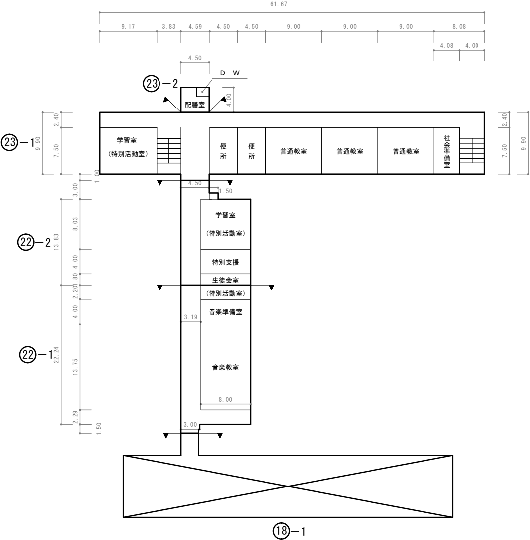
4 階 平 面 図
