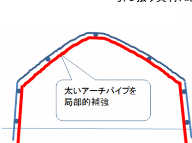
引っ張り資材による肩部補強の参考例
