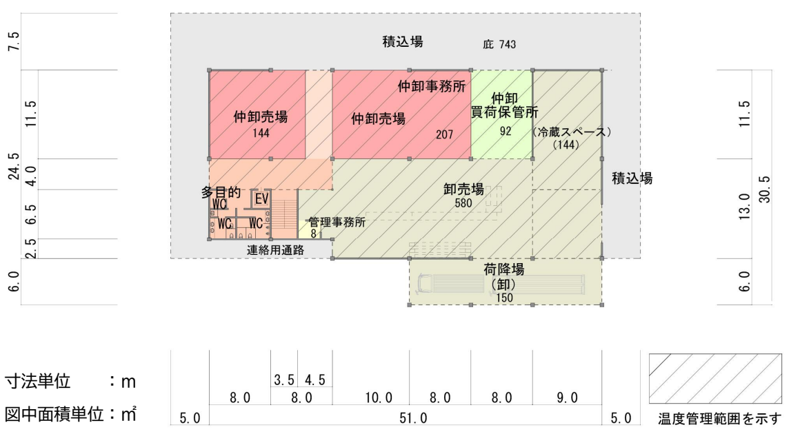
花き棟 1階
