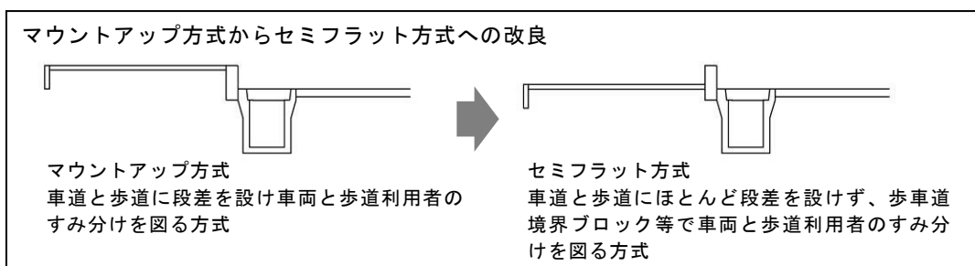
▲マウントアップ方式とセミフラット方式の模式図（再掲）
