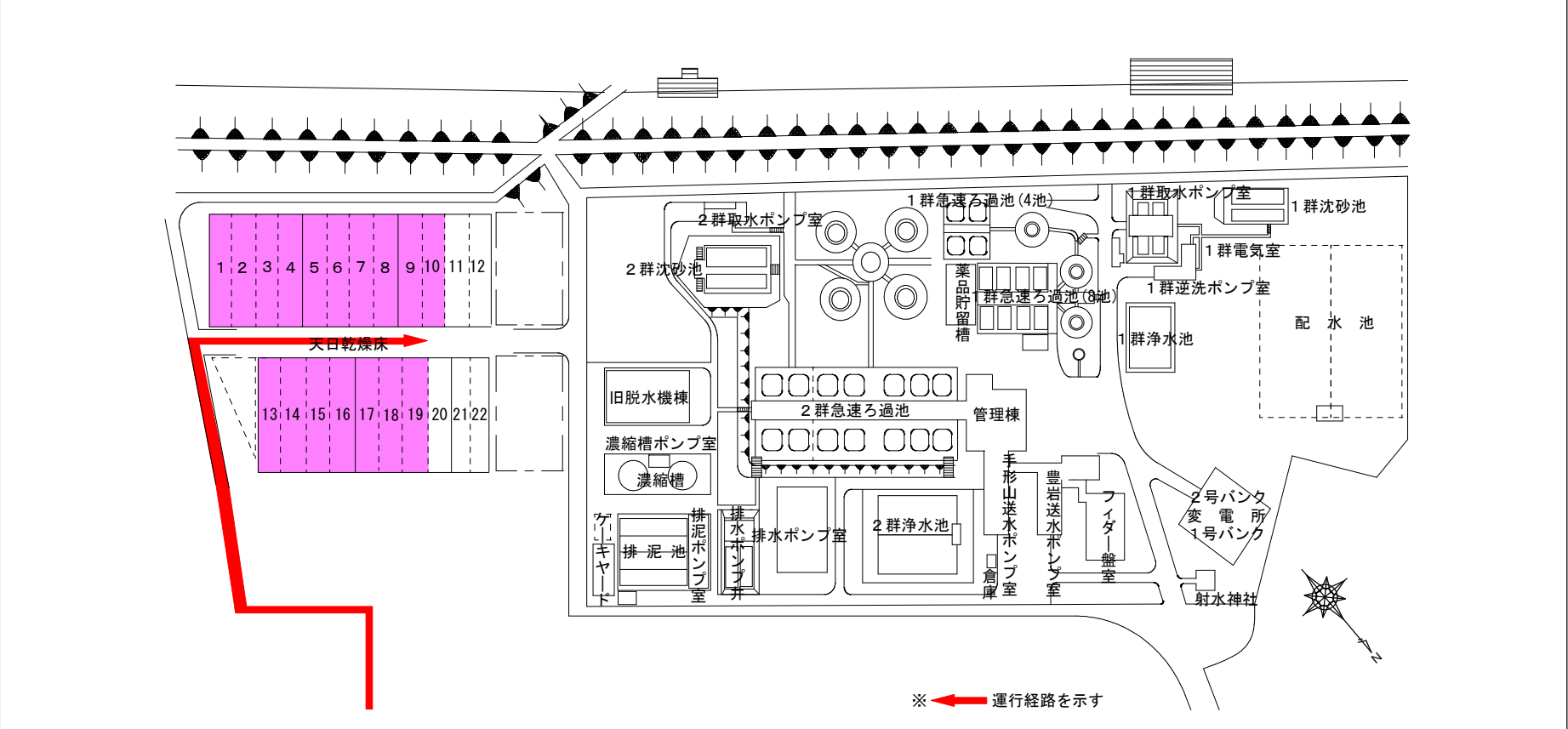
仁井田浄水場配置図 S=1/2,000
