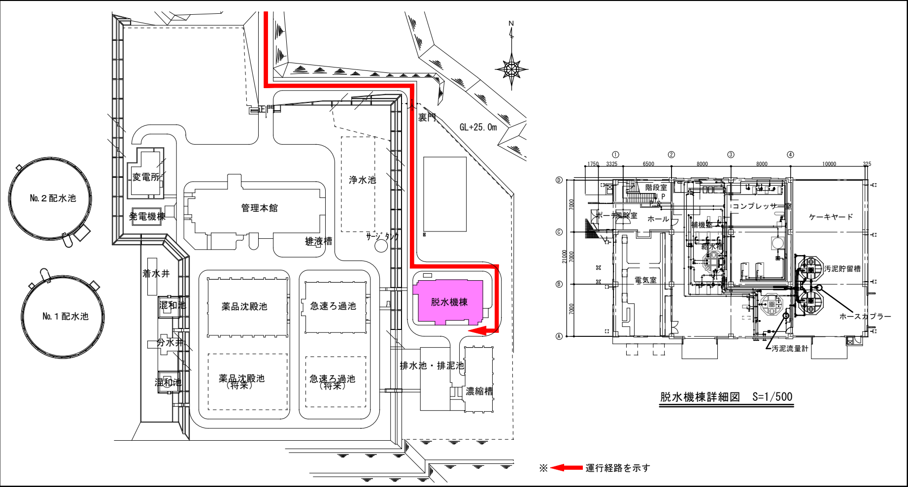
豊岩浄水場配置図 S=1/2,000
