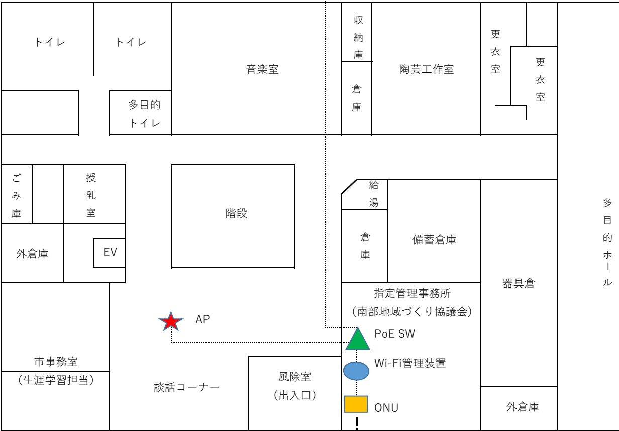
1 階平面図
