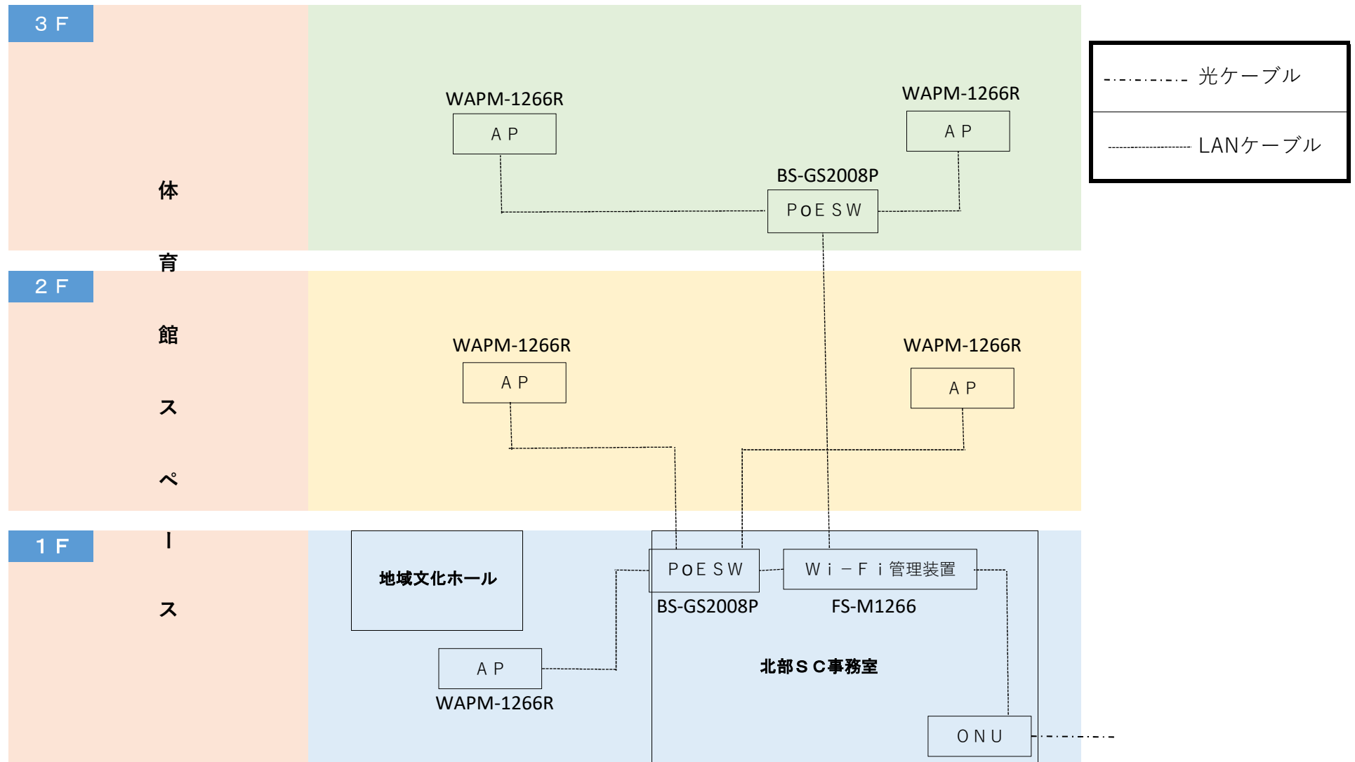
北部市民サービスセンター（機器配置図）
