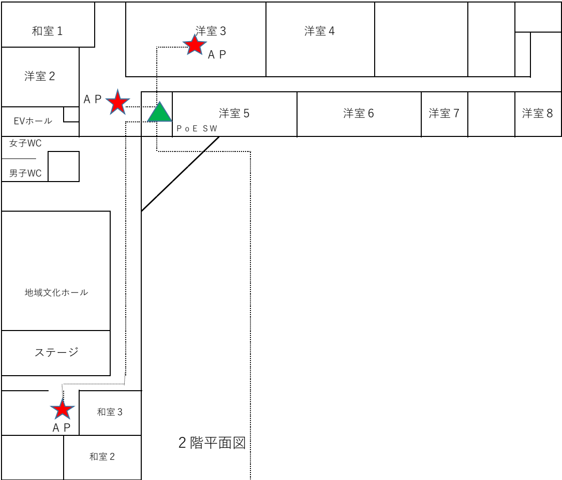
雄和市民サービスセンター（施設平面概略図）
